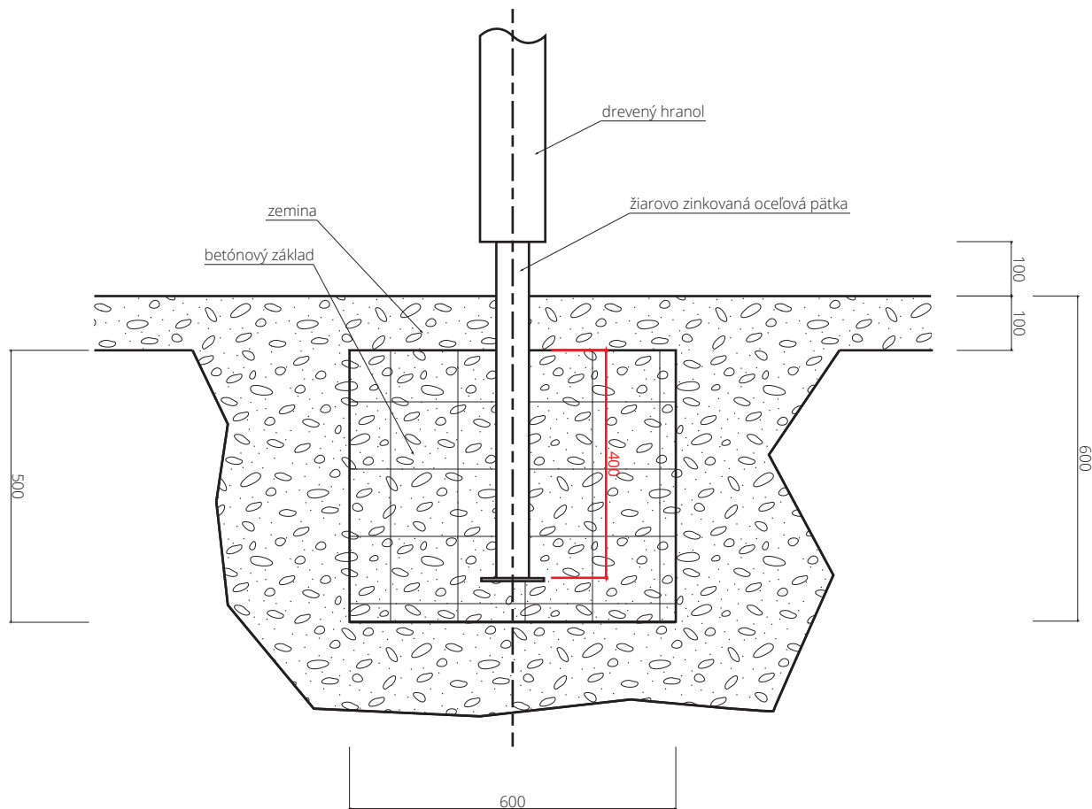
Detail ukotvenia
